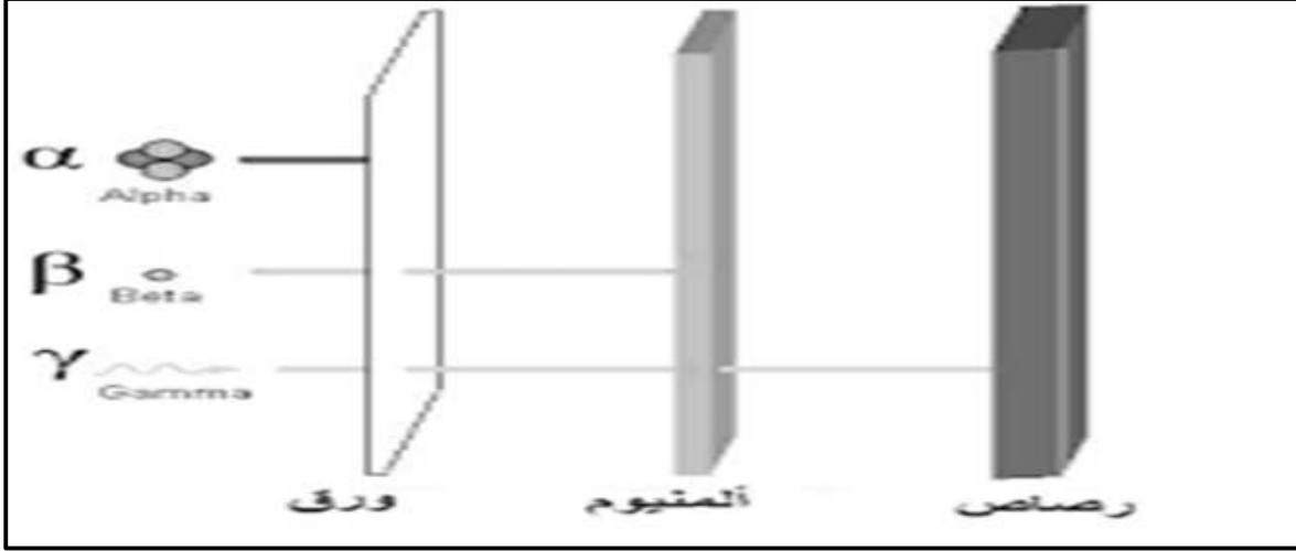
الشكل رقم (٣) يوضح قدرة اختراق بعض الاشعاعات للمادة
